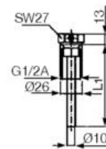
G1/2" menetes csatlakozás 10 mm átmérő. Modell: TW998
