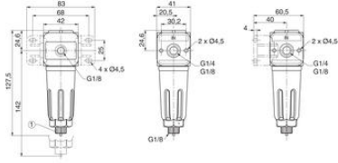
① Semi-automatik dränring, anslutning G1/8*
