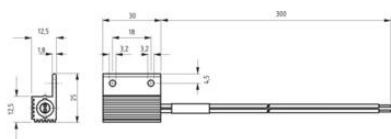
Thermostat KTO 011 (NC)
